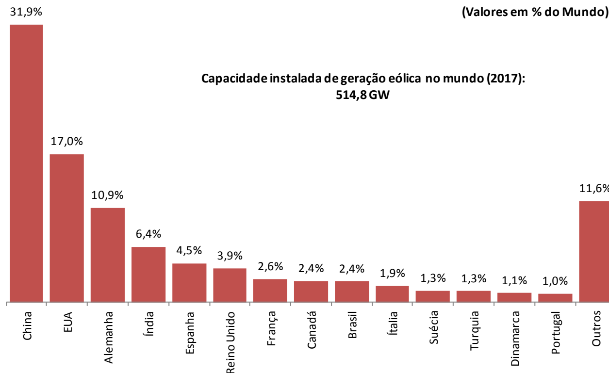
Gráfico 7 - Capacidade instalada mundial de geração eólica - 2017
