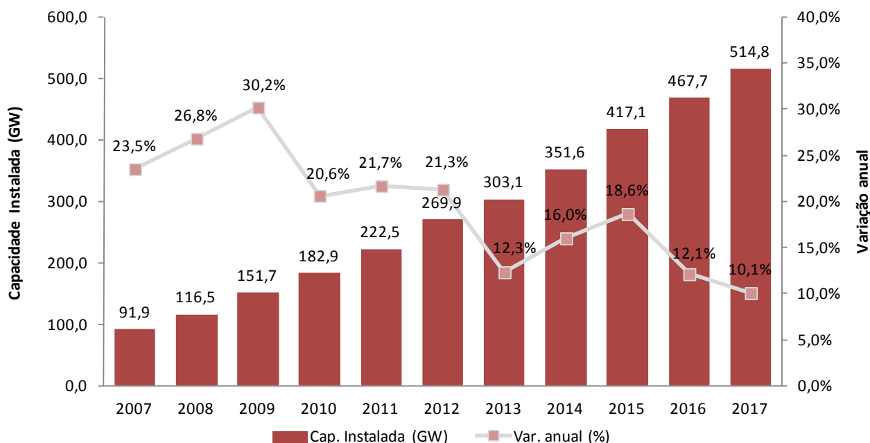
Gráfico 6 - Evolução da capacidade instalada de geração eólica no mundo (GW)
