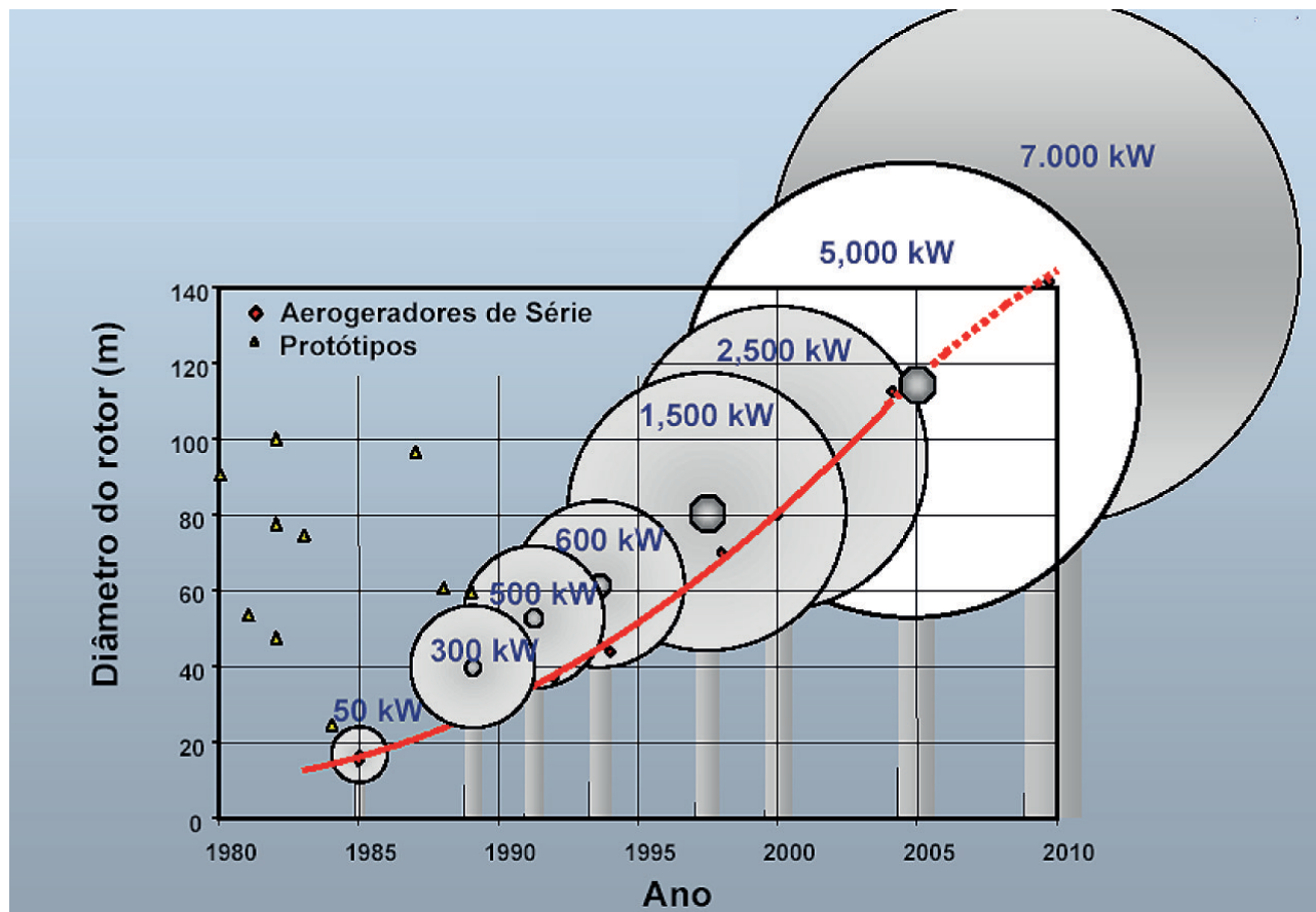
Figura 2 – Evolução da potência de aerogeradores
