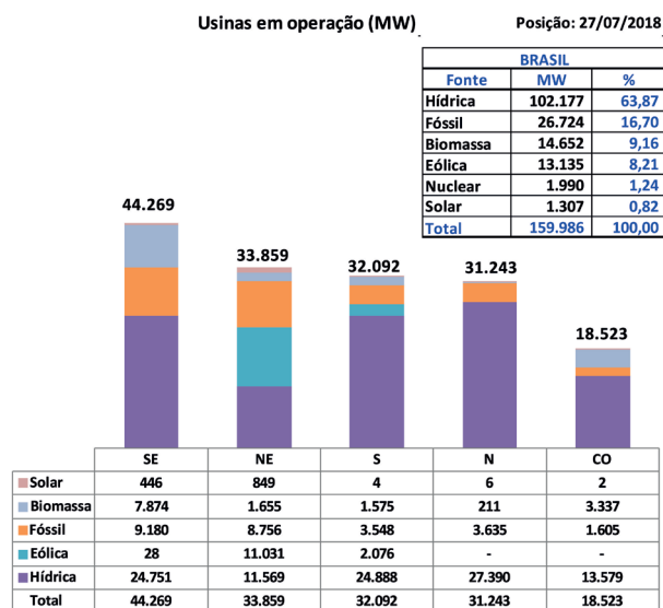
Gráfico 1 – Brasil e regiões: potência instalada de geração de energia elétrica por fonte
