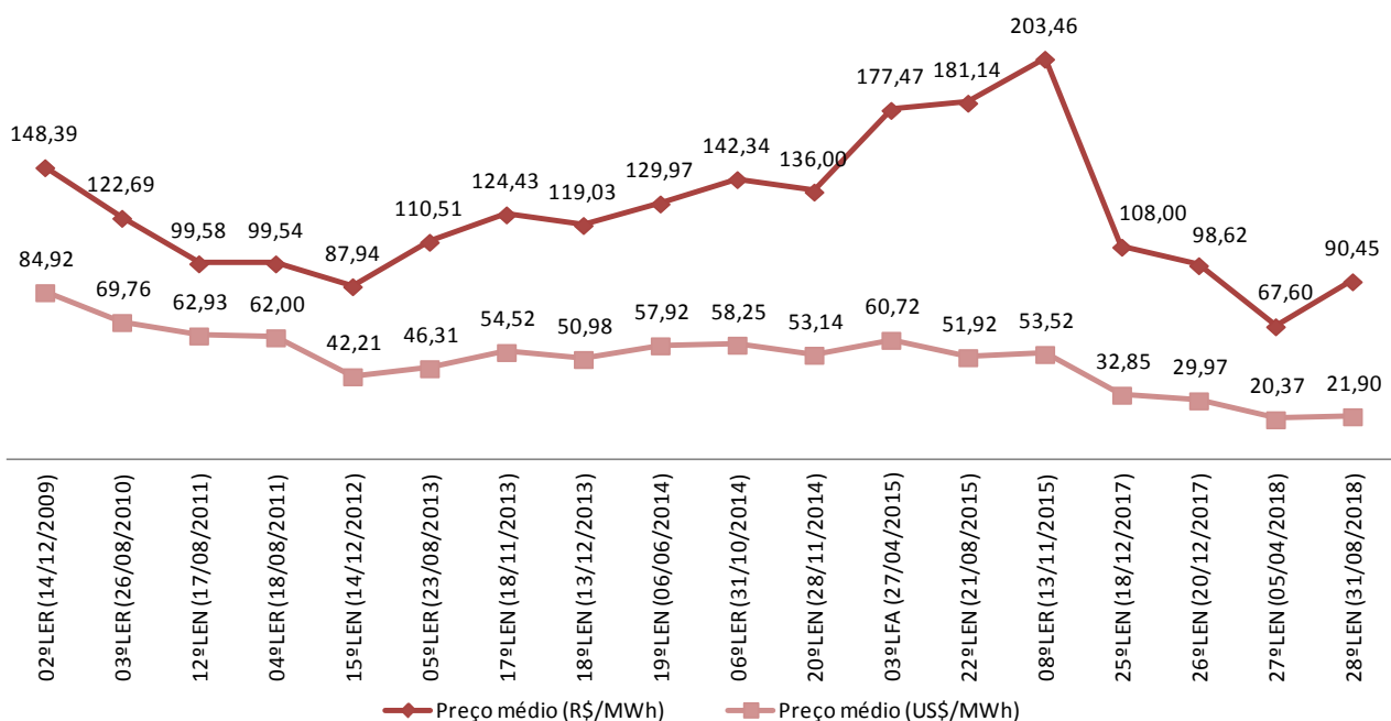
Gráfico 11 – Preços médios dos projetos eólicos aprovados nos leilões realizados pela ANEEL
