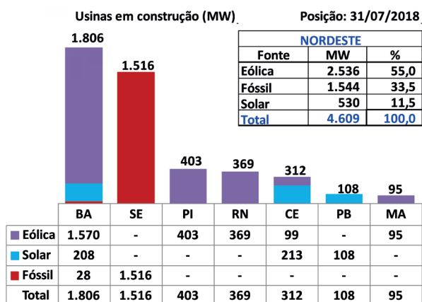
Gráfico 3 – Nordeste: usinas em construção, por fonte e estado da Região
