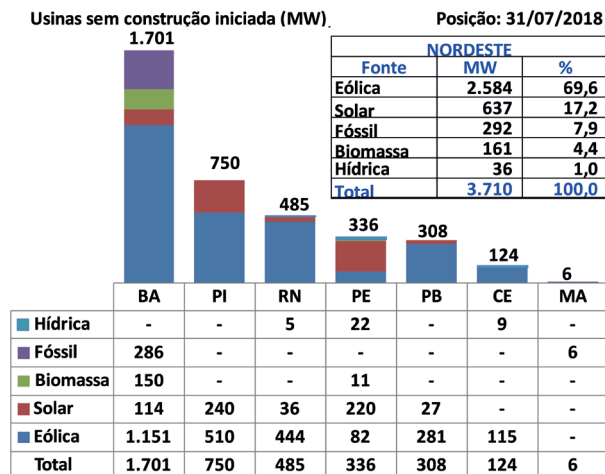
Gráfico 4 – Nordeste: usinas previstas sem construção iniciada, por fonte e estado da Região
