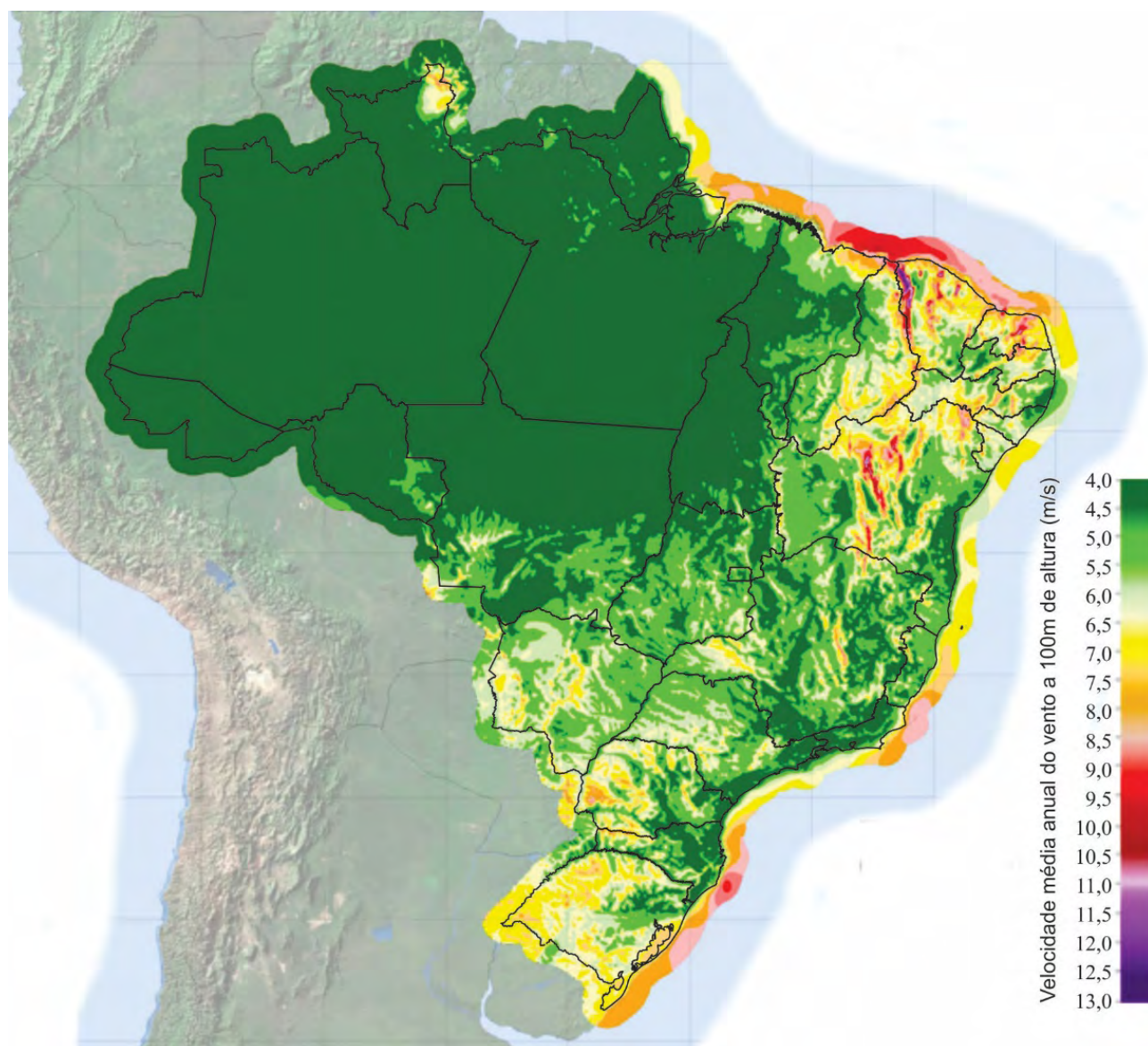
Figura 3 – Potencial eólico do Brasil
