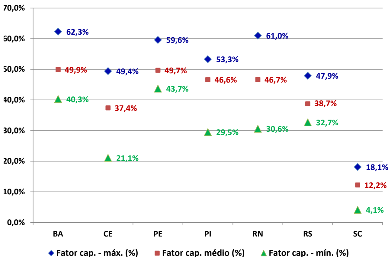
Gráfico 12 – Fatores de capacidade mínimo, médio e máximo verificados em 2017 nos estados
