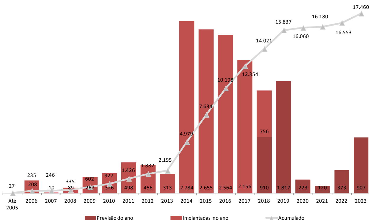
Gráfico 8 – Evolução e projeção da capacidade instalada de geração de energia eólica no Brasil (MW)
