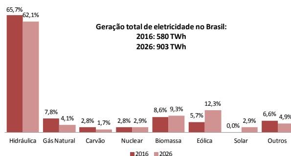
Gráfico 9 – Participação das fontes na geração de energia elétrica do Brasil – 2016 e 2026 (% do total de geração no ano)
