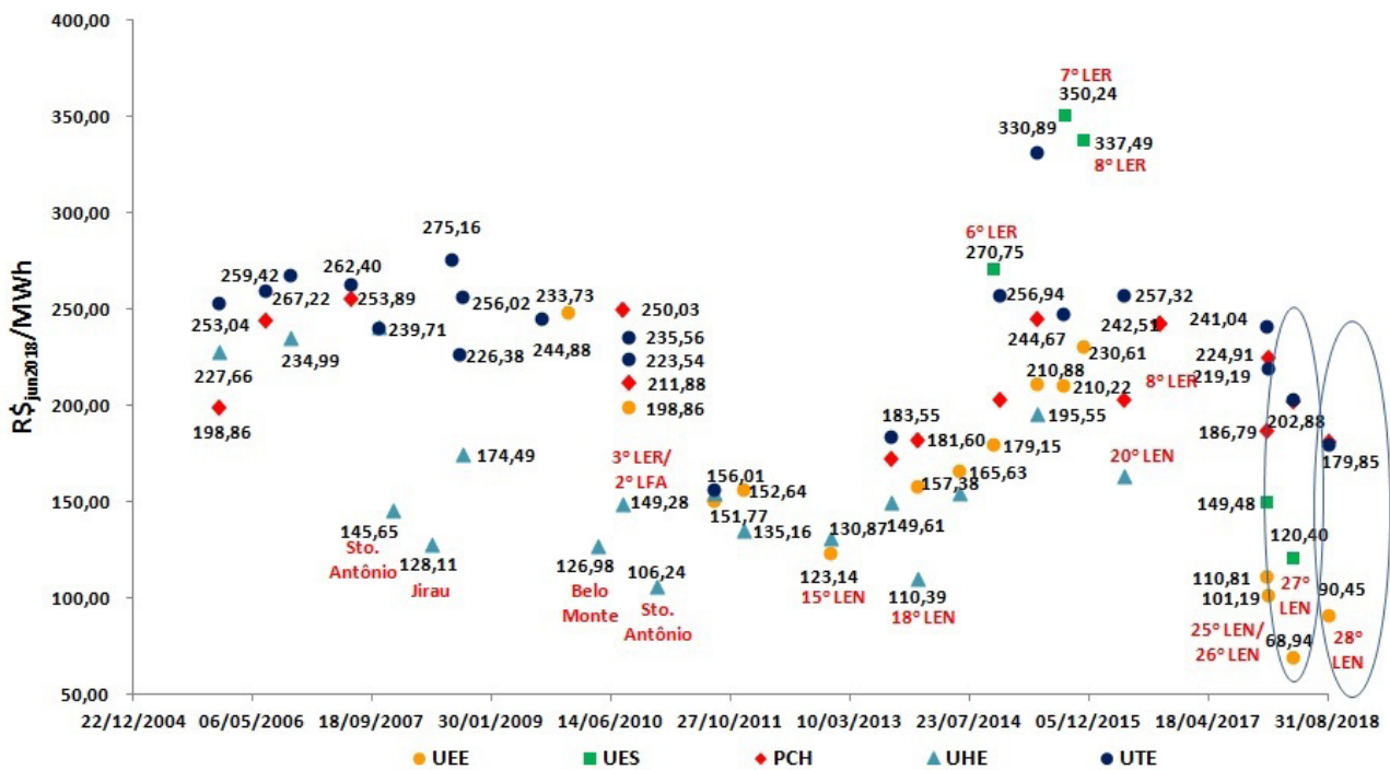
Gráfico 10 – Preço médio por fonte de energia observados nos leilões realizados pela CCEE (R$/MWh – valores constantes de junho/2018*)
