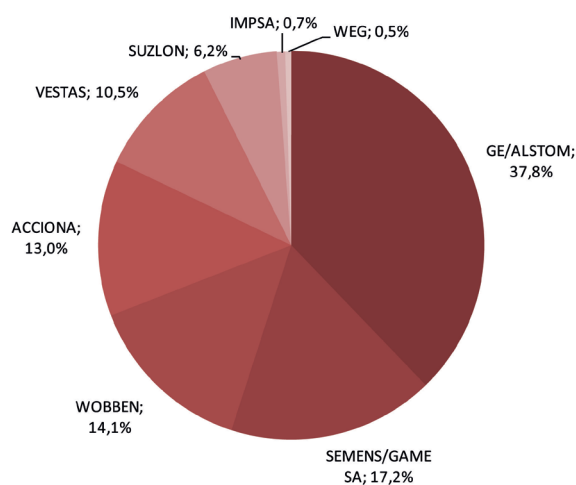
Gráfico 5 – Participação dos fabricantes de aerogeradores nos projetos eólicos em operação no Brasil
